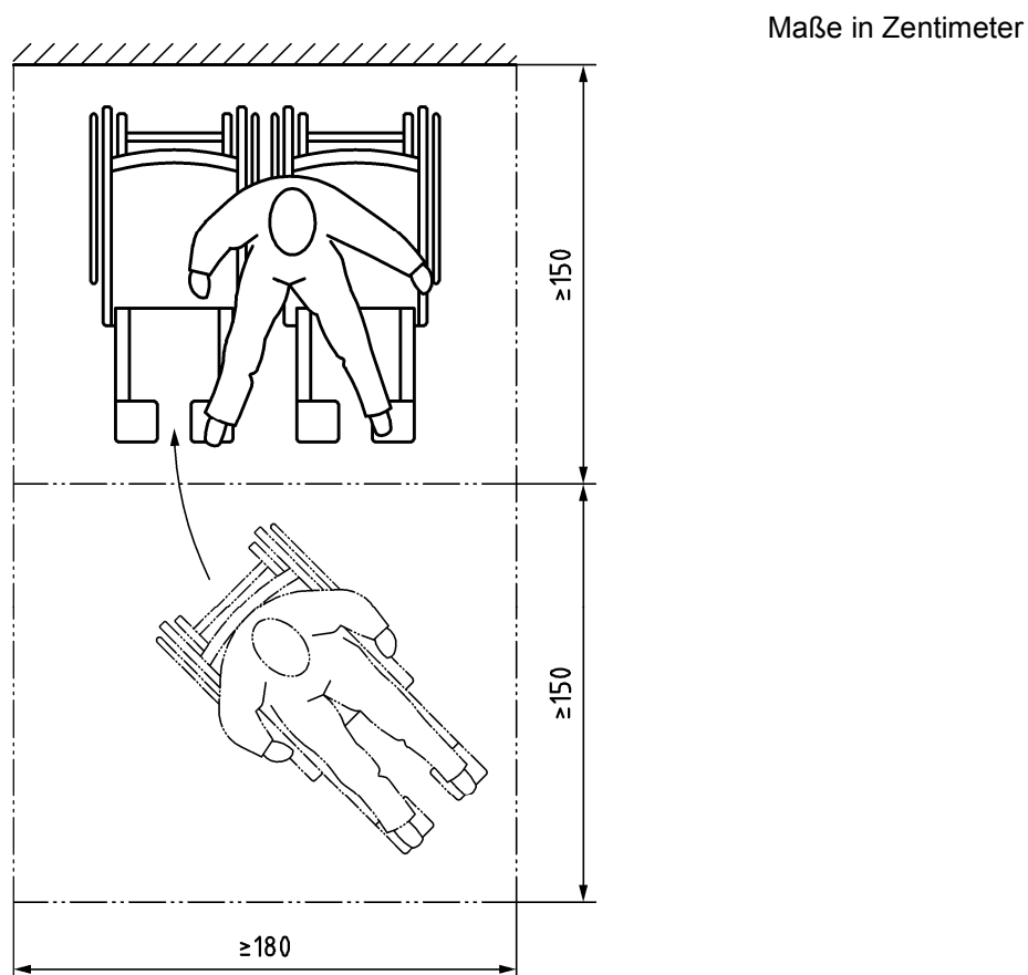
Bild 9 — Platzbedarf für den Rollstuhlabbstellplatz einer Person, Bewegungsfläche für Rangieren und Wechsel
