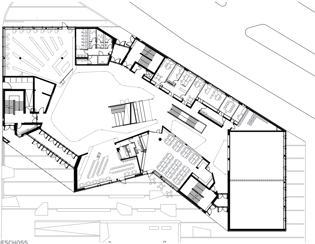
GRUNDRISS ERDGESCHOSS
